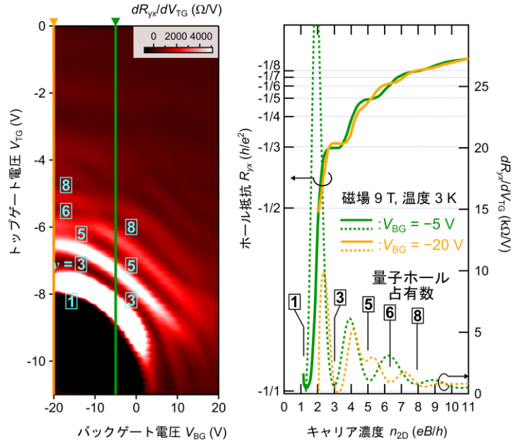
図 3. トポロジカル半金属 (\text{Cd}_{1-x}\text{Zn}_x)_3\text{As}_2 薄膜 ( x = 0.7 、膜厚 75 nm) においてデュアルゲートによる量子ホール効果のマッピングを行った結果（左）と、代表的なバックゲート電圧（緑：-5 V と黄：-20 V）における、トップゲート電圧 V_{TG} 掃引に対するホール抵抗 R_{yx} と一階微分 dR_{yx}/dV_{TG} の変化（右）。ワイル軌道が存在する場合に予測されるストライプ状の量子ホール伝導度が観測されている。
