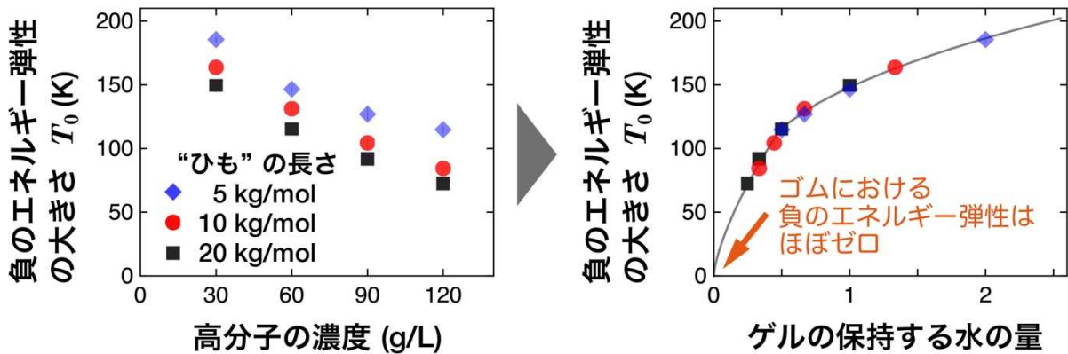
図3：「負のエネルギー弾性」の背後にあるシンプルな物理法則。左図のように、負のエネルギー弾性の大きさ（図2の T_0 ）は、ゲルにおける高分子の網目構造（高分子の濃度および網目を構成する“ひも”の長さ）に応じて様々な値を取る。本研究グループは、負のエネルギー弾性の大きさが、右図のようにシンプルな物理法則に従うことを明らかにした。右図の横軸は、「ゲルの保持する水の量」を表す。横軸の値がゼロになると、水を保持しない「ゴム」に対応する。ゲルの保持する水の割合を減らしてゴムに近づけると、負のエネルギー弾性の大きさがゼロに近づく。この結果は、「ゴムのやわらかさはエントロピー弾性でおおむね決まる」という100年近い長年の先行研究ともつじつまが合う。
