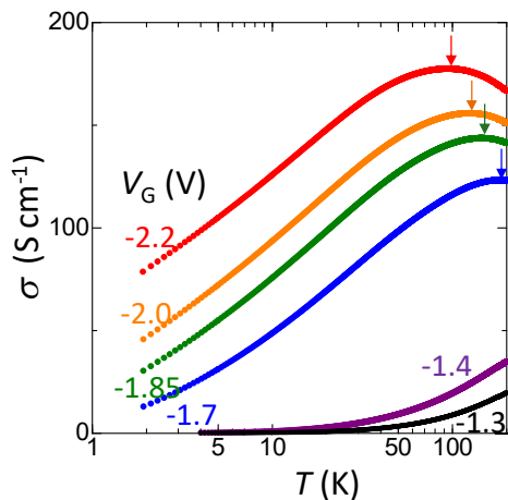
図3 PBT TT膜の高ドープ下での電気伝導率 \sigma の温度依存性
