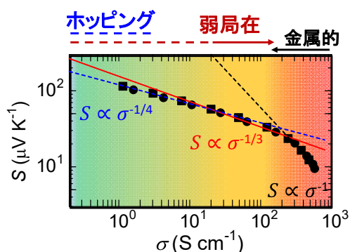
図6 PBTIT 膜の室温でのゼーベック係数の電気伝導率依存性
