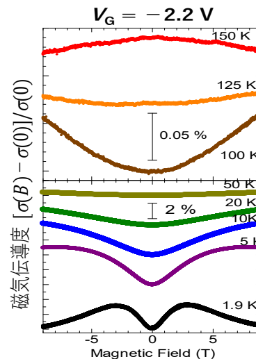
図4 PBT TT膜の最大ドープ時の磁気伝導度の温度依存性 （横軸は磁場）
