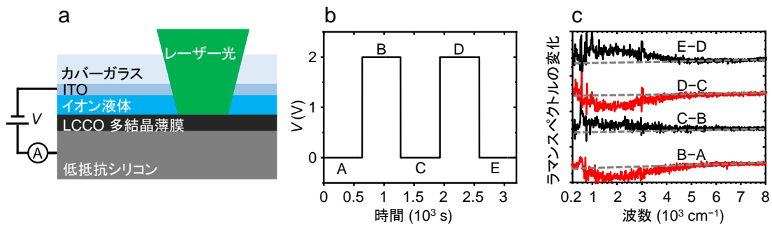
図2. (a) ラマン分光用試料の断面図。電圧印加下のマグノンの変化をレーザー光で調査するために、透明導電膜であるITOを上部電極として用いた。(b) 印加電圧の時間依存性。(c) 電圧印加及びショートによるラマンスペクトルの変化。A-Eの記号は(b)のそれに対応している。~2000 \text{cm}^{-1} を中心とする幅広い変化がtwo-magnonピークによるものである。
