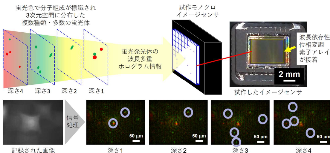
図 2 上段：ホログラフィックカラー多重 3 次元蛍光顕微鏡応用の実験と試作したイメージセンサ。 下段：実験結果。丸印内は合焦された蛍光体
