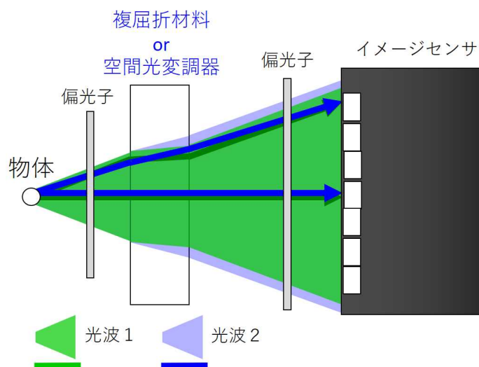
インコヒーレントデジタルホログラフィの記録光学系の一例
