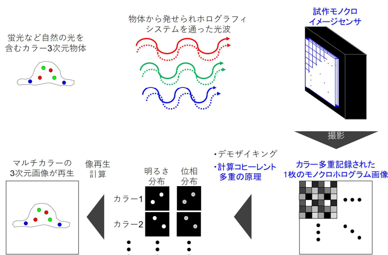
図 1 今回開発したセンシングシステムの測定手順
