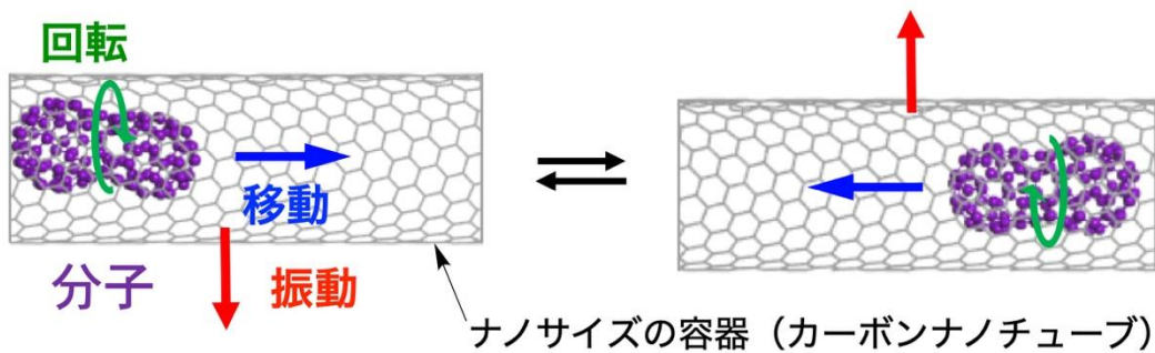
図1：我々の目に見えるマクロスケールの世界では、マラカスを振ると中の小石がその振動にตอบสนองして（力学的応答）回転しながら容器の中を動く。本研究では上述の高速電顕動画撮影を用いて、ナノ（微小）スケールの器である CNT の中に閉じ込めた分子が、CNT の振動にตอบสนองして CNT の軸に沿って往復運動をすることが見いだされた。
