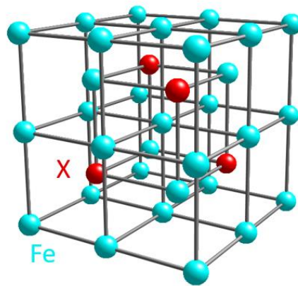
図5 Fe_3X ( X = Ga, Al )の結晶構造。青色が鉄、赤色がガリウム（またはアルミニウム）を表します。
