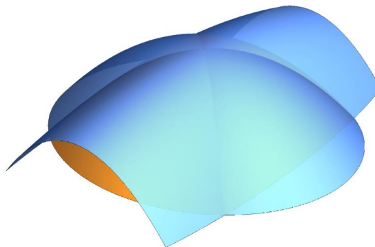
図6 ノーダルウェブの概念図。十字に走っているライン上で青色と黄色の面（バンド）が
