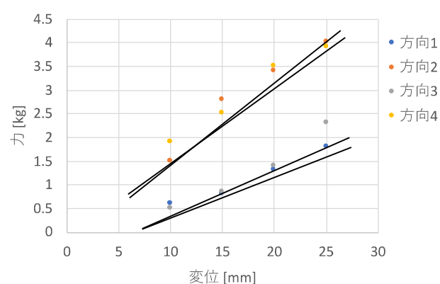
図3 作業支援用リム先端剛性係数
