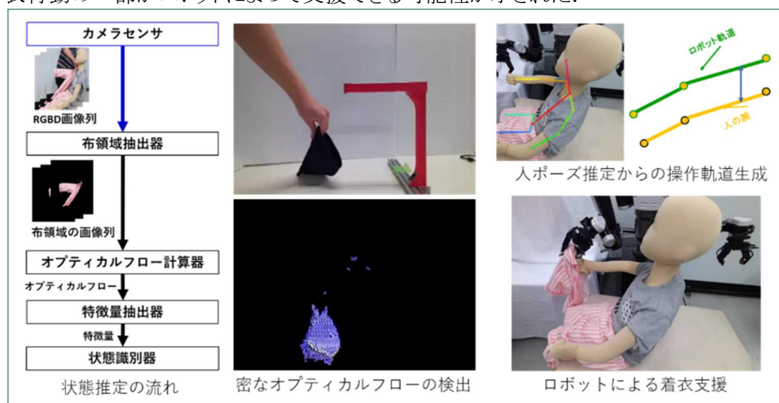
図1 布状態推定手法の全体像
