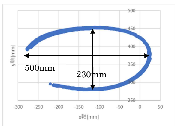
図2 作業支援用リム先端軌道
