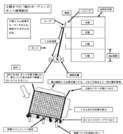
庁舎ネット設計図 設計・製造・設置すべて職員で行いました。
