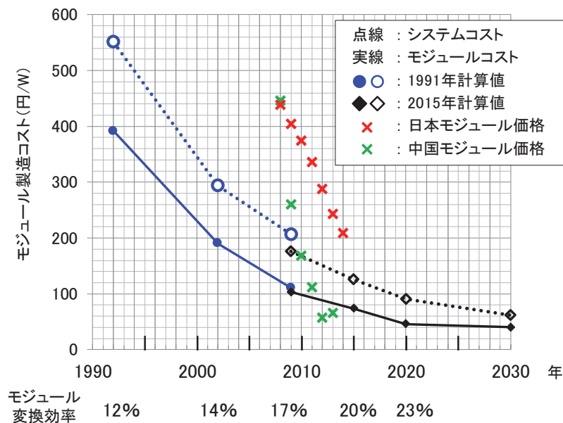
図 3 モジュール製造コストの計算値と実勢価格の比較
