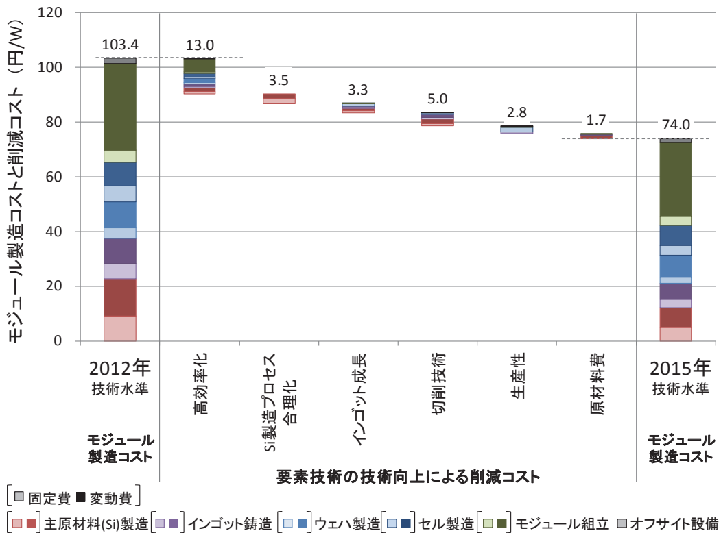
図 2 単結晶シリコン太陽電池モジュール製造コストとコスト削減技術 (製造工程別、固定費・変動費によるコスト構造)
