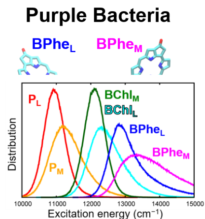
図6. 紅色細菌の反応中心内の色素の励起エネルギーの分布。
