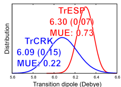
図 1. TrCRK 法での遷移双極子モーメント計算は、TrESP 法で計算したものより大幅に改善した。
