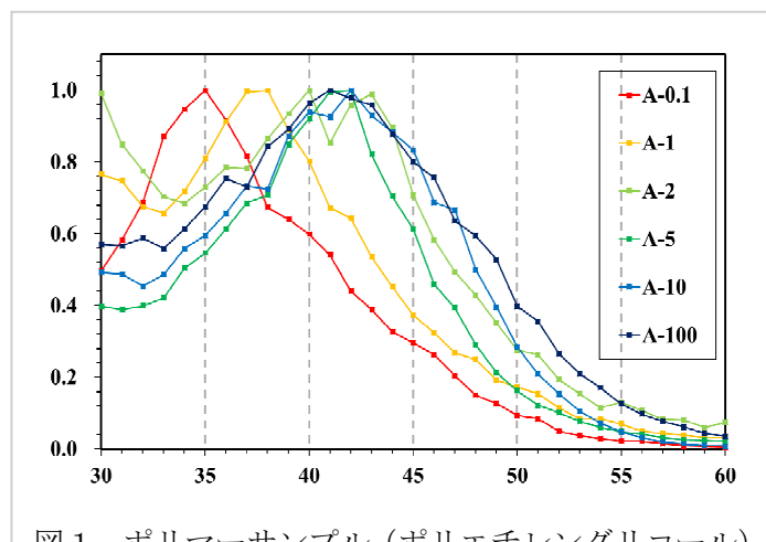
図1. ポリマーサンプル（ポリエチレングリコール）に添加剤（クエン酸）を加えた際の分子量分布の変化。縦軸は分布の最大値を1として規格化したもの、横軸は重合度を表し、系列名の添え字（0.1, 1 など）は高分子に対する添加剤のモル比を表す。
