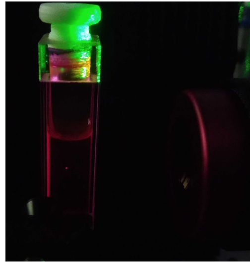
図 1: パラメトリック光によるローダミンからの2光子蛍光
