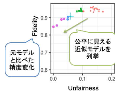
図 2：説明モデル列挙の例 (Adult income データの場合)
