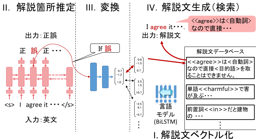
図 2: あいまい検索を応用した解説文生成
