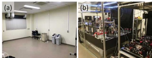
図1：新規実験室の整備。(a) 本研究課題開始時。(b) 2020年12月現在の様子。手前が自作レーザー冷却光源系、奥が超高真空チャンバー系。
