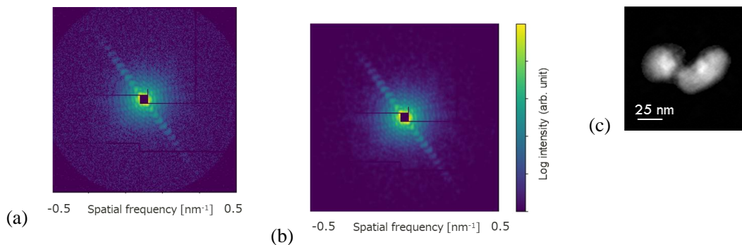
図 5 SACLA BL2 にて計測したナノ粒子からのコヒーレント回折パターンと再構成試料像。 (a) 二種類のナノ粒子の混合試料からのコヒーレント回折パターン (b) (a)のノイズ除去データ (c) 混合試料の再構成試料像
