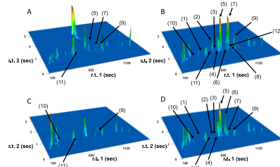
図3. 3次元ガスクロマトグラム (A) (C) 雄を誘引しない雌から生じる匂い物質 (B) (D) 雄を誘引する雌から生じる匂い物質
