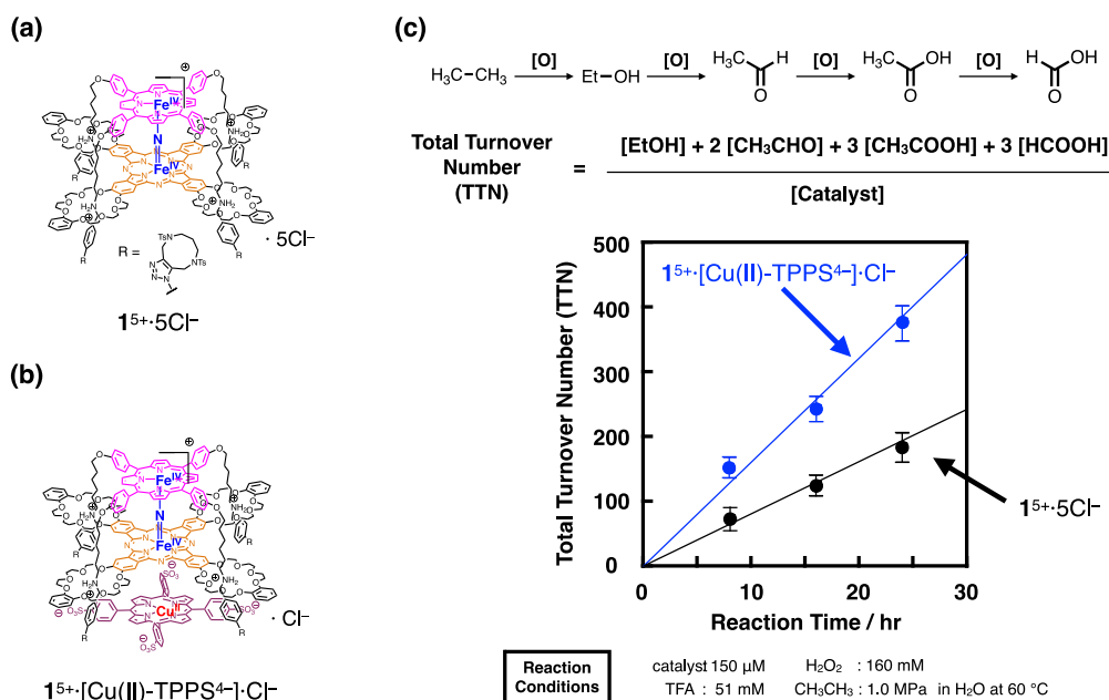
Fig. 1 (a) 15^+\cdot 5\text{Cl}^- および(b) 15^+\cdot [\text{Cu}(\text{II})\text{-TPPS}_4^+]\cdot \text{Cl}^- の構造と、(c) 15^+\cdot 5\text{Cl}^- 、 15^+\cdot [\text{Cu}(\text{II})\text{-TPPS}_4^+]\cdot \text{Cl}^- を用いた触媒的エタン酸化反応の結果。
