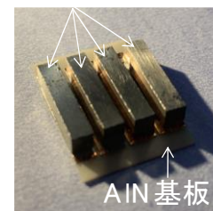
Co_2MnGa 焼結体 ( 15 \times 3 \times 3 mm^2 )
