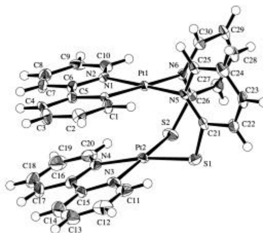
図 1. syn-[Pt 2 (pytd) 2 (bpy) 2 ] 2+ の構造
