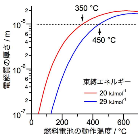
図14 プロントラッピングモデルに基づいて計算した、燃料電池の動作に必要なプロトン伝導が得られる温度と電解質の厚さの関係
