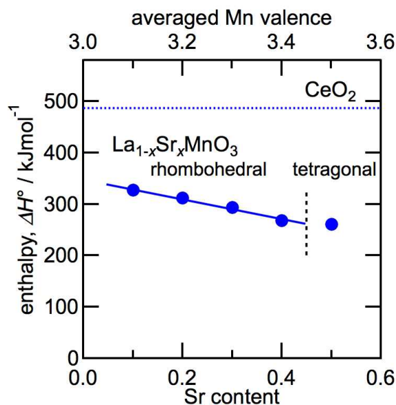
図6. ストロンチウム添加 \text{LaMnO}_3 における酸化還元エンタルピーのストロンチウム濃度依存性
