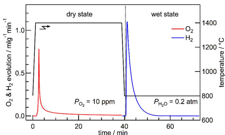
図2 \text{La}_{0.8}\text{Sr}_{0.2}\text{MnO}_{3-\delta} を用いた熱化学水分解の一例(熱サイクル:1400–800℃)
