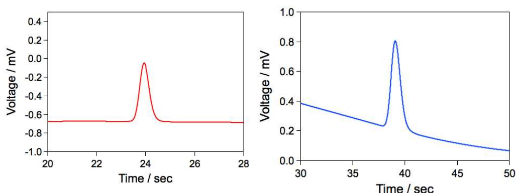
図7 \text{La}_{0.6}\text{Sr}_{0.4}\text{MnO}_{3-\delta} による \text{O}_2 および \text{CO} 生成時のクロマトグラム
