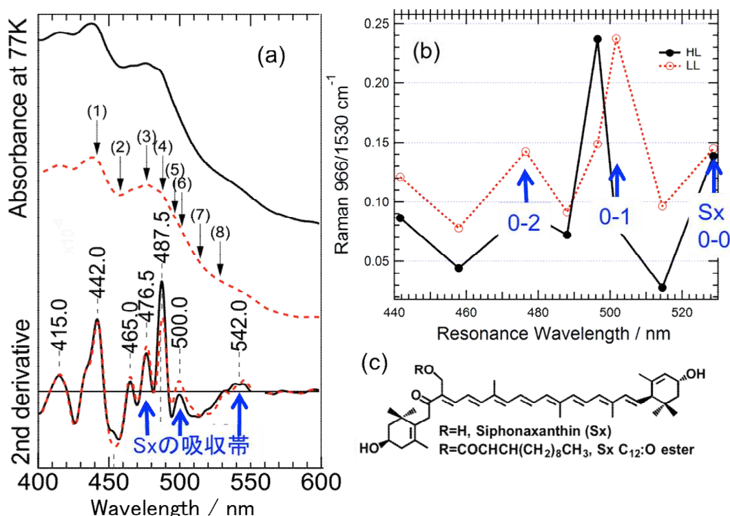
図3 (a)モツレミル系状体の77Kにおける吸収スペクトル及びその二次微分スペクトル、(b)カロテノイドの面外変角振動を示す \mu ラマン線の励起波長依存性(高照度:黒実線、低照度:赤点線)、(c)シフォナキサンチンの化学構造式。これらにより帰属したシフォナキサンチン(Sx)の吸収帯(0-0、0-1、0-2遷移)を矢印で示した。SCP はルテインがシフォナキサンチンに置換され、LHCII におけるルテインと同様に、生体内における機能単位である三量体構造の要となっていることが示唆された。[文献 5. (1) 3 より改変]
