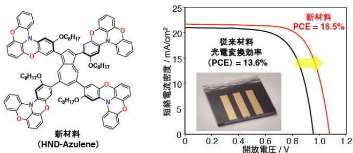
Fig. 5. 座布団型有機半導体材料とペロブスカイト太陽電池特性.
