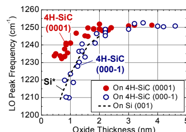
図6. 成長した熱酸化膜をエッチバックして薄膜化したときの Si-O-Si 伸縮振動 LO モードのピークシフト。結晶面による違いが見られる。参考のため、Si 基板上の熱酸化膜の文献データ(*S. Miyazaki et al., Appl. Surf. Sci. 113/114, 585 (1997))を点線で示した。
