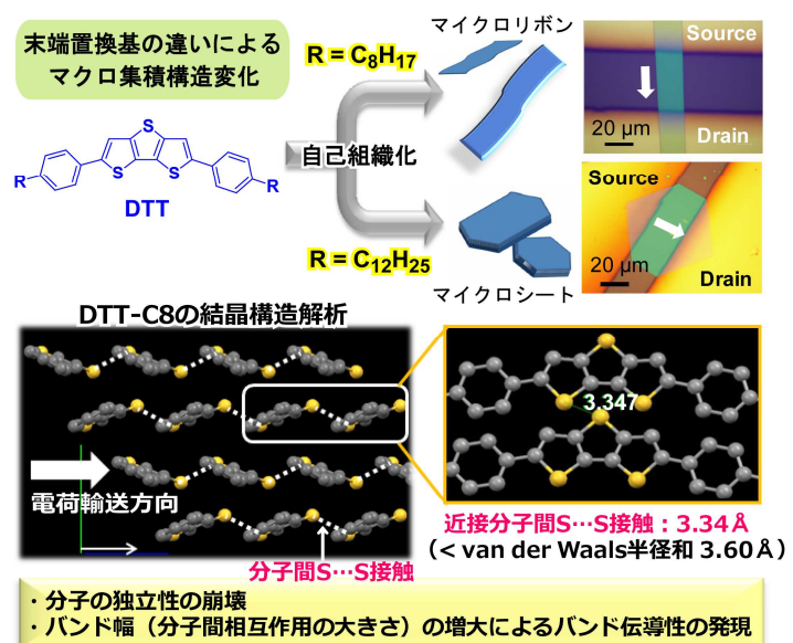
図1 DTT 誘導体によるマイクロリボン・シート形成(上)と特異的分子集積に基づく高効率電荷輸送機能の発現(下)
