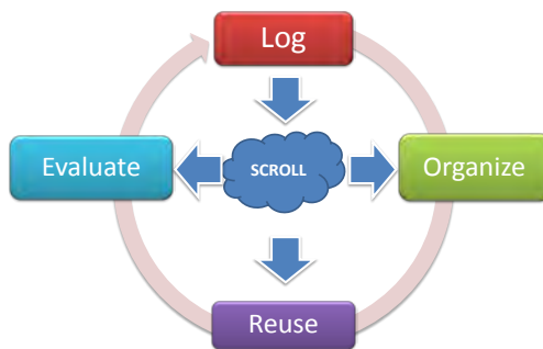
図1: LORE モデル
