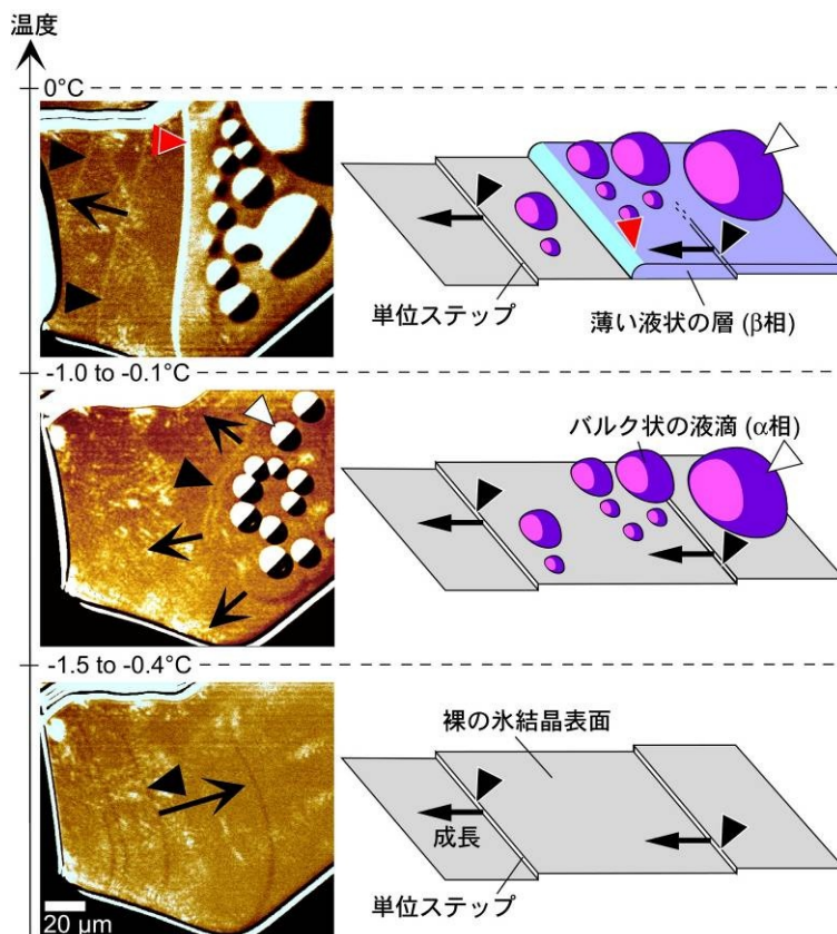
図3 氷結晶の六角底面上で生成する2種類の表面液体相。図の左側は光学顕微鏡写真で、右側は模式図。 \alpha 相 (白三角) と \beta 相 (赤三角) の発生温度は実験のたびに若干のずれを示したが、同じ実験中では常に \beta 相は \alpha 相よりも高温で発生した。2種類の表面液体相は、ダイナミックに氷結晶表面上を動き回り、合体を繰り返した。黒三角は氷結晶表面上の水1分子高さの分子層 (単位ステップ) を示す。
