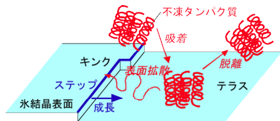
図1 氷結晶表面での不凍タンパク質の挙動と、それに対する氷結晶の分子層(その成長端をステップと呼ぶ)の応答。
