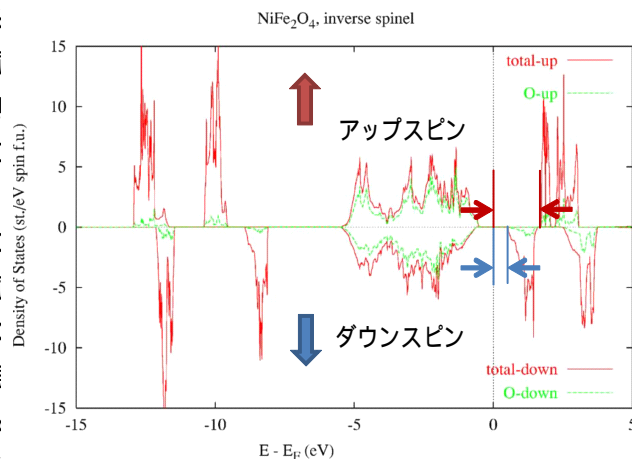
図5 \text{NiFe}_2\text{O}_4 の電子状態密度。Z. Szotek et al. , Phys. Rev. B 74, 174431 (2006)
