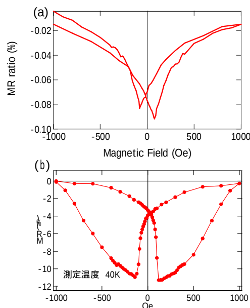
図 4 スピンフィルター接合の磁気抵抗効果。(a) \text{MgO}(001)/\text{Fe}_3\text{O}_4(50\text{nm})/\text{NiFe}_2\text{O}_4(4\text{nm})/\text{AlO}_x(2\text{nm})/\text{Fe}(20\text{nm}) スピンフィルター接合。測定温度は室温。(b) \text{MgO}(001)/\text{TiN}(50\text{nm})/\text{Fe}_3\text{O}_4(4\text{nm})/\text{AlO}_x(2\text{nm})/\text{Fe}(20\text{nm}) スピンフィルター接合。測定温度 40K。
