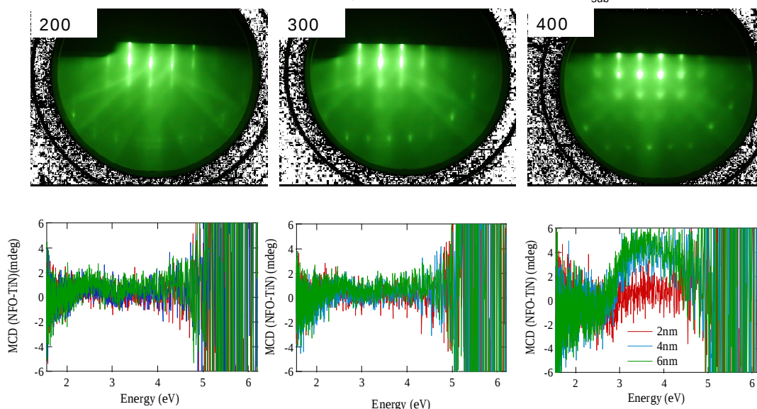
図3 \text{MgO}(001)/\text{TiN}/\text{NiFe}_2\text{O}_4(2,4,6\text{nm}) 膜の各成長温度での RHEED 像及び各膜厚での磁気光学効果。
