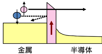
図 1 スピンフィルターの概念図。上向きスピンのみを通し、下向きスピンはね返す。
