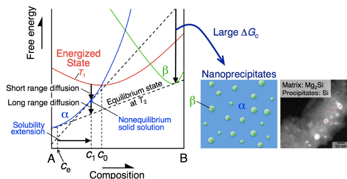
図 3. A-B 二元系の自由エネルギー模式図．"energized state" は，MA 後の非平衡状態である． \alpha 相の自由エネルギー曲線の勾配が大きければ (ラインコンパウンド等)，過飽和固溶体を得るため高いエネルギーが必要である一方，平衡状態
