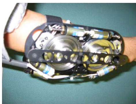
図3 回転モーメント型運動方向提示デバイス
