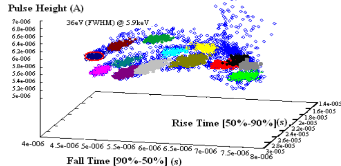
20ピクセルIr-TESアレイ素子とX線(6keV)入射波形弁別による入射ピクセル別信号分布
