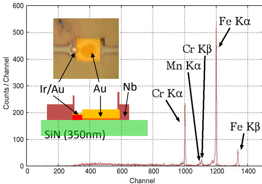
放射線吸収領域/超伝導温度センサ分離型TES素子によるステンレス蛍光X線元素分析スペクトル(Spring-8 BL01B1)
