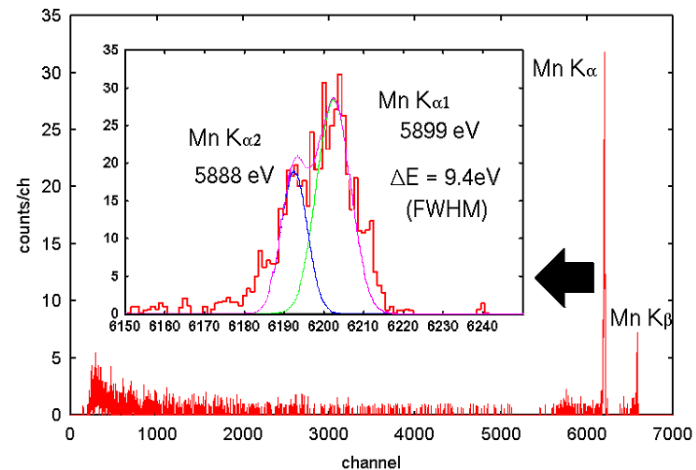
Ir/Au近接2重層TESによる ^{55}\text{Fe} 線源からのX線エネルギースペクトル
