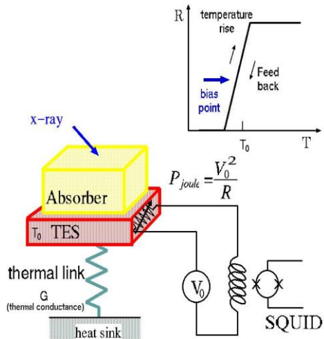
超伝導転移端センサ(TES)概略図
