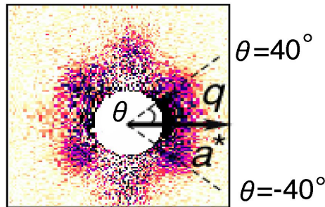
図3 : 中性子小角散乱データ。(H ext =0, T=1.6K) \theta = \pm 40^\circ 付近に磁束格子の存在を示す散乱が観測されている。 測定がゼロ磁場下で行なわれているため、弱強磁性の内部磁場により形成された自己誘起磁束格子構造の存在を示す。
