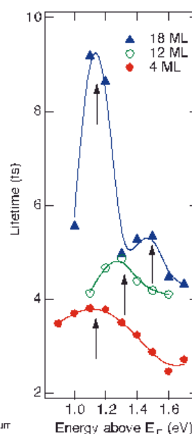
図3 寿命
