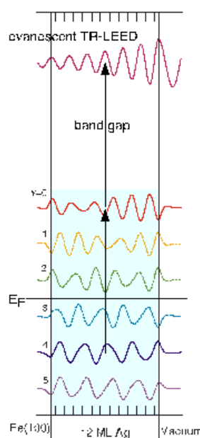
図2 波動関数
