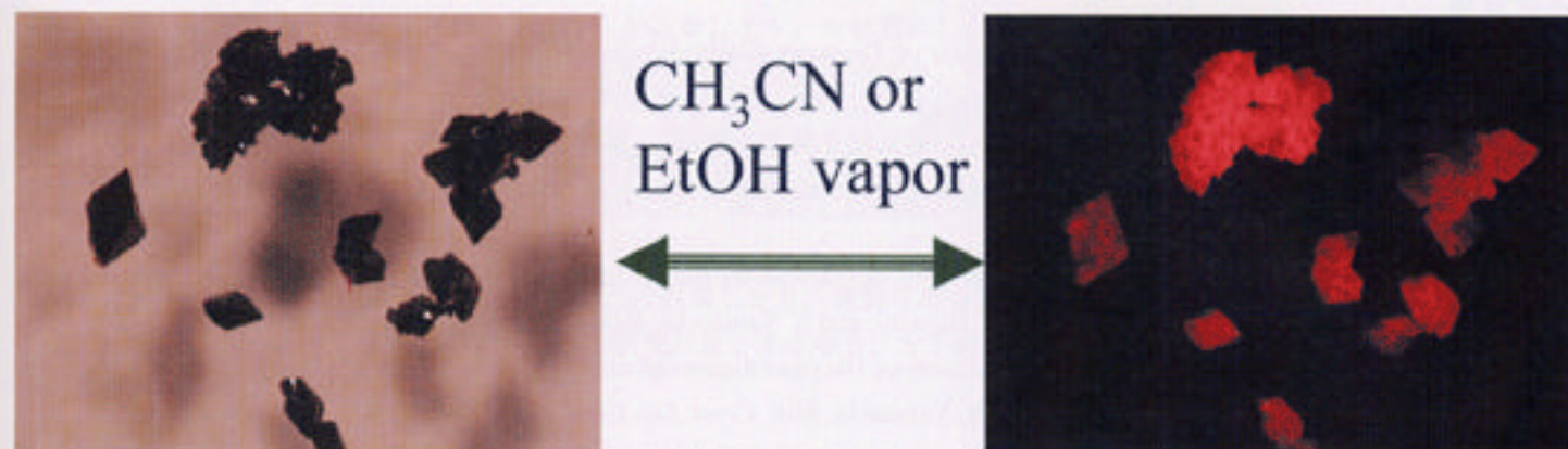
図1 syn型 [Pt(py)_2(bpy)](PF_6)_2 結晶におけるベイボクロミズム
