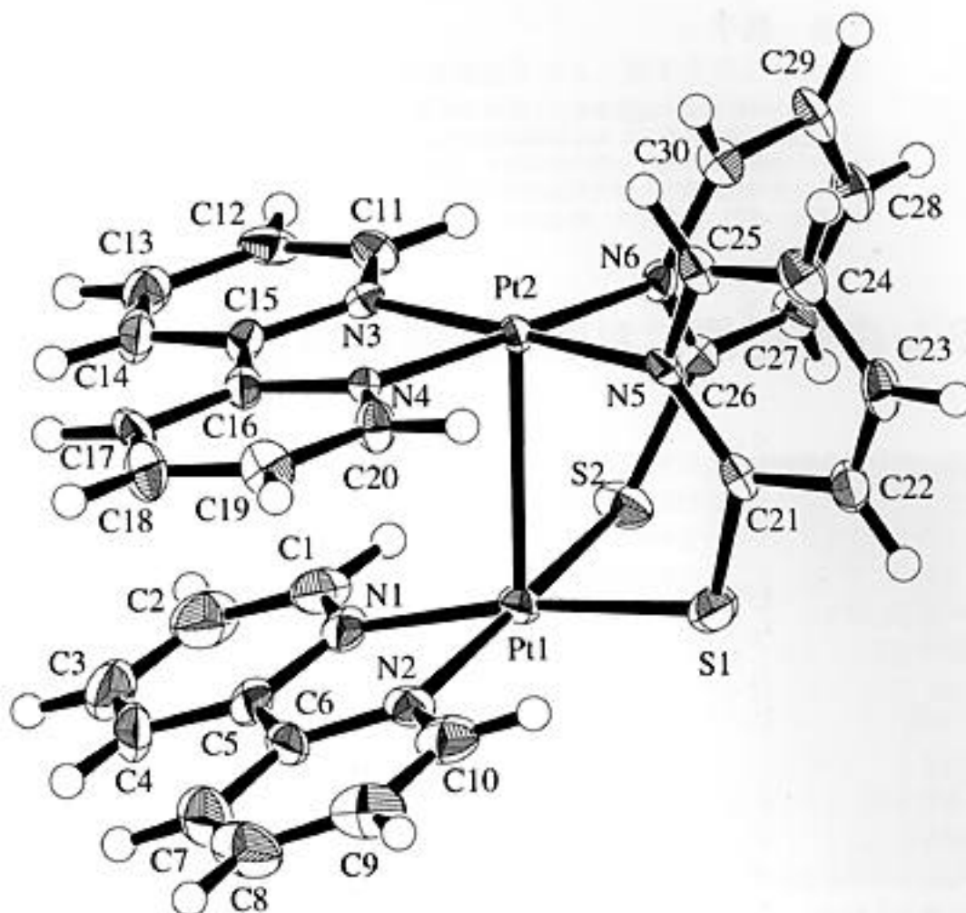
図2 syn型 [Pt(pyt)(bpy)] 2+ の構造
