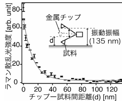
図1: CNT の近接場ラマン散乱の銀ナノ探針-CNT 間距離依存性
