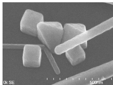
図2: ポリオール法により合成した銀ナノ構造(立方体、双三角錐およびロッド)の電子顕微鏡像。
