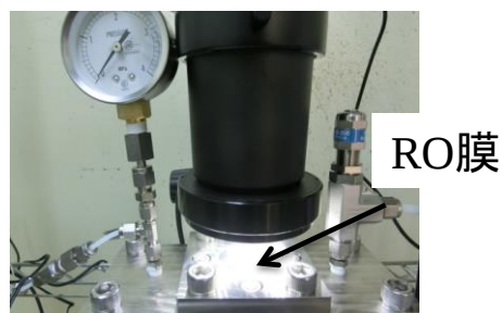
図5-1 RO膜上のバイオフィーム・ バイオフィーリング抑制試験装置 □
