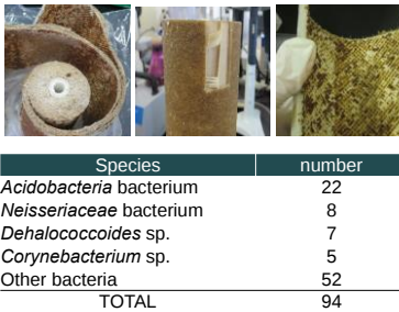
図 1-4 ファウリングを起こした RO 膜の菌叢解析図
