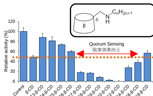
図 1-5 アルキルアミノ化 \beta -CD による S. marcescens AS-1 株の QS 阻害
