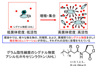
図1-1 微生物コミュニケーション (Quorum Sensing)
