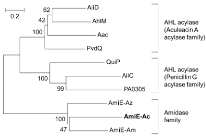
図 1-3 AmiE の系統解析図
