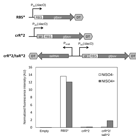
図 7 リボレギュレーターの模式図および Synechocystis sp. PCC 6803 中での機能確認
