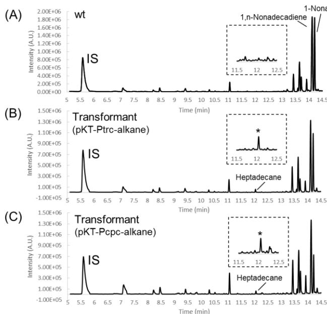
図 12 アルカン合成遺伝子導入 Synechococcus sp. NKBG 15041c における炭化水素生産の評価 (A) 野生株、(B) pKT-Ptrc-alkane 保持株、(C) pKT-Pcpc-alkane 保持株
