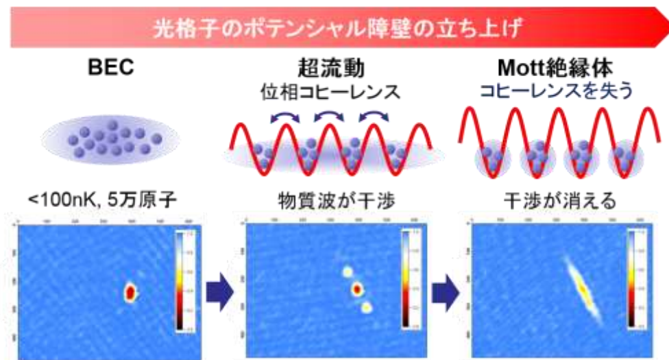
図 5: 光格子における超流動-Mott 絶縁体相転移。トラップから原子集団を解放し、15ms 自由拡散させた後に原子の吸収像を撮像した。
