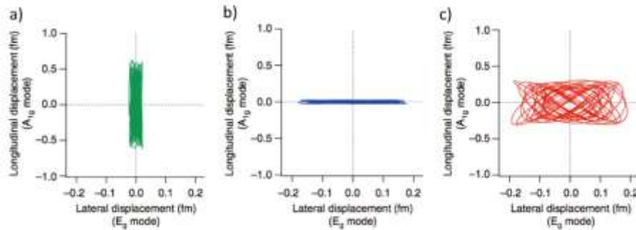
図8: ビスマス固体内の原子の2次元運動の制御。(a)パルス間隔49.4fs (b) 92.2fs (c) 93.6fs (H. Katsuki et al. , Nature Commun.4, 2801 (2013).)
