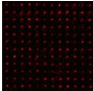
図 7: 顕微システムを用いたナノホールサンプルの透過光イメージ。直径約 100nm のナノホールアレイ(2.5 \mu m 間隔)から成るサンプルを利用し、顕微システムの分解能評価を行い回折限界に近い約 800nm の分解能を得た。図は電荷増幅型 CCD カメラで撮像したサンプルのイメージである。なお、サンプルは分子科学研究所の飯野教授、京都大学の横川准教授より提供して頂いた。
