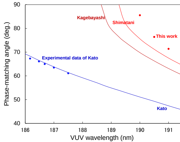
図26 189nm 光近傍の位相整合角度 (CBO)
