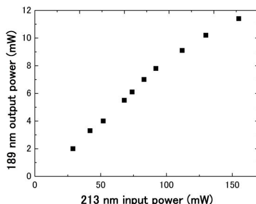
図27 189nm 光出力特性 (15mm CLBO、室温)
