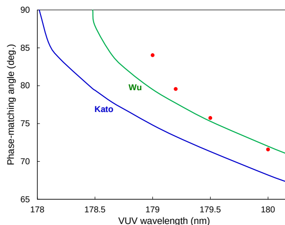
図23 179nm 光近傍の位相整合角度 (LBO)
