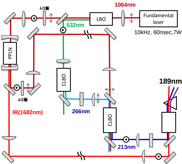
図24 189nm 光発生用光学系
