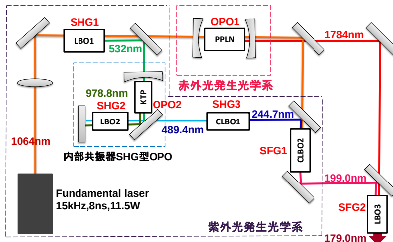
図21 179nm 光発生用光学系
