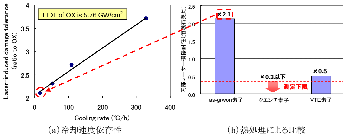
図4 CBO 結晶の 355nm 紫外光レーザー損傷耐性比較(1-on-1)
