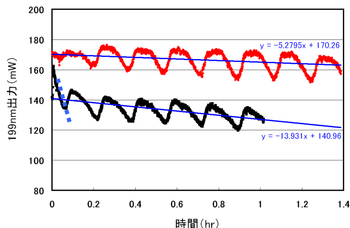
図16 199nm 光発生評価結果(赤線:開発結晶素子、黒線:従来素子)
