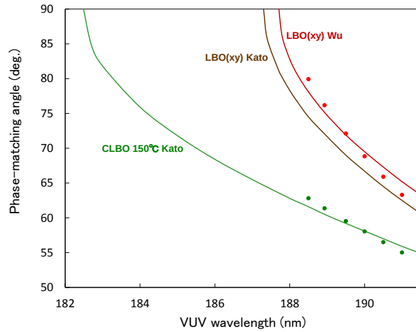
図25 189nm 光近傍の位相整合角度 (LBO、CLBO)
