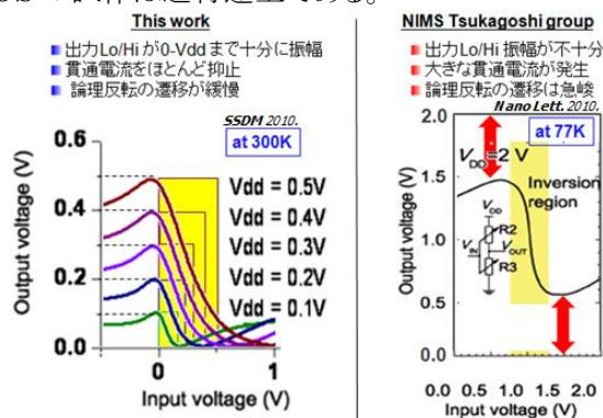
図 4.4.4 左 : GOSFET による CGOS インバータ動作(A. Moutaouakil et al, SSDM J3-4, 2010.)。トップゲートによるしきい値制御は施していない。Vdd を-0.5 V から+0.5 V までの範囲内で論理反転動作が
