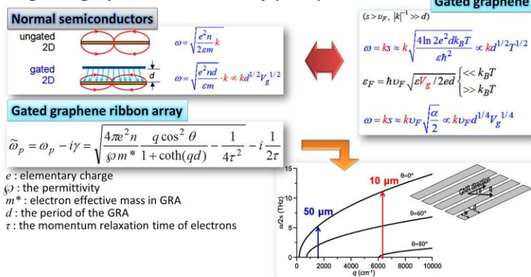
図 4.3.4 ゲーテッドグラフェンおよびグラフェン・ナリボンにおけるプラズモンの分散特性[26]。
