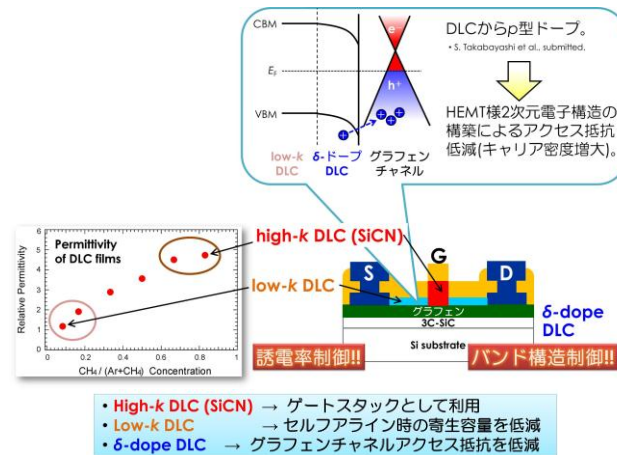
図 4.2.8 DLCによる機能性絶縁膜。DLC内不純物 \delta ドーピングによるグラフェンへのキャリアリモートドーピングのイメージ(上)。成長雰囲気内 \text{CH}_4 濃度による DLC 誘電率の制御(左下)。ゲートスタックへの High-k DLC、パッシベーションへの Low-k DLC の適用と \delta ドーピング DLC とによる高性能 GOSFET 開発戦略(右下)。
