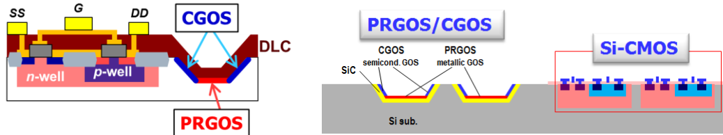
図 8.2 CGOS-PRGOS-CMOS 完全モノリシック LSI 断面図（バックエンドプロセス前）。
