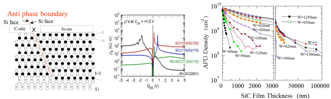
図 4.1.12 グラフェン/3C-SiC/Si の基板リークパス。左：逆位相境界欠陥（APBD）の断面図。中：各種面方位の GOS と 6H-SiC(0001)上にエピ成長したグラフェン試料の比抵抗を厚みで規格化して比較（3C-SiC エピ層厚は 200nm 固定）。膜厚で規格したバルク比抵抗 \rho_B と比較すると、GOS 基板の 3C-SiC 抵抗率は 6H-SiC 基板の最低値（ <10^{-1} k \Omega m）よりはむしろ高い。右：逆位相境界欠陥（APBD）の 3C-SiC 膜厚ならびにパターンサイズの依存性数値解析結果。 \mu m オーダーに 3C-SiC を厚膜化することで、基板電流リークの 2 桁程度の低減が推定される。
