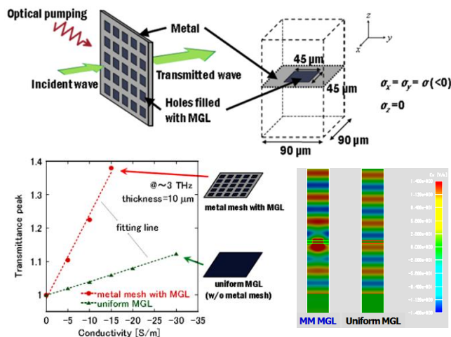
図 4.3.11 光学励起によって反転分布状態におかれたグラフェンに金属メッシュ構造を施した場合に得られるテラヘルツ波透過励における利得増強効果。単純平面グラフェンに比して高い増幅効果が得られる。[50, 74]
