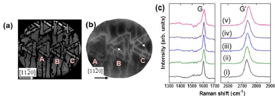
図 4.1.11 μGOSにおける三角形に形成したエピタキシャルグラフェン：EGの形成領域サイズに対する結晶品質の依存性[72]。(a) LEEM 像。一辺 5μm のパターン A では表面平坦性が高い。一辺 6μm, 7μm のパターン B, C では平坦性が劣化している。(b) PEEM (光電子顕微鏡) 像。多層グラフェンは白く見える。一辺 5μm のパターン A は単層グラフェンのみ。一辺 6μm, 7μm のパターン B, C では多層グラフェンが領域内に含まれる。(c) Raman スペクトルの EG 形成領域サイズ依存性。(i)から(v)の順にそれぞれ、限定なし、一辺 7, 6, 5, 4 μm。いずれのスペクトルも欠陥に起因する D バンドピーク(～1360 cm -1 )が皆無であり、結晶品質が高いことを表わしている。G'ピークのシフトより、形成領域サイズの縮小化とともにグラフェンと SiC の格子定数差に起因した圧縮歪が増大していることがわかる。
