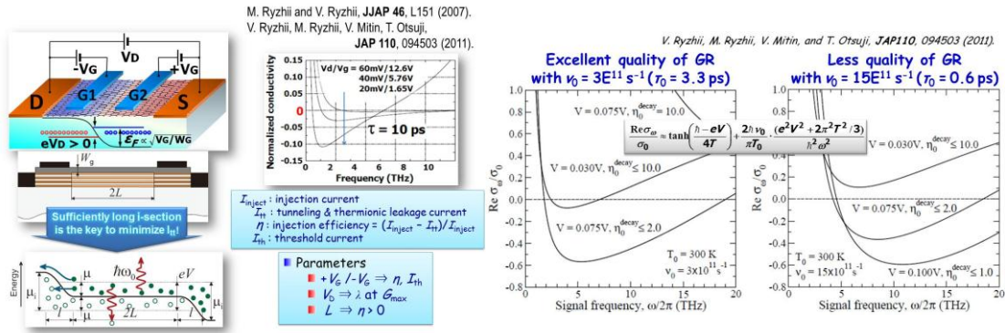
図 4.3.8 デュアルゲート GOSFET 構造による電流注入型グラフェンテラヘルツレーザ。素子構造断面図およびバンド図（左）[25, 60]、ドレインバイアス V_d 、ゲートバイアス V_g をパラメータとして導電率特性第一近似解析結果（左中）[25]、右：デュアルゲート GOSFET 構造による電流注入型グラフェンテラヘルツレーザの高精度モデルに基づく導電率特性解析結果。光学フォノンのエネルギー緩和速度因子（熱伝導度因子）： \eta_0^{decay} を導入し、熱伝導（放熱）特性に対する依存性も明らかにしている。キャリアの運動量緩和時間を高品質、中品質グラフェンを想定し、各々3.3ps（左）、0.6ps(右)を仮定している[60]。
