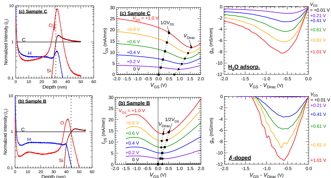
図 4.2.9 DLC 堆積前の水素アニール条件と DLC 堆積中の酸素濃度変調による酸素不純物の DLC 中への \delta ドーピングとそのチャネルリモートドーピング効果。上：DLC/グラフェン(SiC)界面に酸素不純物が偏析した結果、酸素不純物からの正孔リモートドーピングによってグラフェンチャネルが p 型 (Dirac 電位が正にシフト) 特性を示す。下：酸素不純物が DLC/グラフェン界面から DLC 内に 3 nm 入った位置に \delta ドーピングされている。その分、上図に比してキャリアリモートドーピング効果が低減され、Dirac 電位は 0 V に接近。同一キャリア濃度での電界効果移動度は、酸素が DLC/グラフェン界面に偏析した上図に比して高く。HEMT の効果が得られている。ドレイン電流変調能力を表す相互コンダクタンス： g_m は、ゲート絶縁膜厚が 1.5 倍厚いにもかかわらず、 \delta ドーピング効果によって 1.4 倍以上に向上している。ゲート絶縁膜厚で規格化すると \delta ドーピングによる増大は 200%以上になる。
