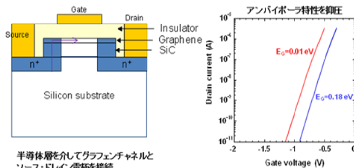
図 4.4.6 グラフェン層から SiC と Si 基板を介してソース・ドレインコンタクトを取る構造によりアンバイポーラ特性を回避できるソース・ドレイン構造の構造図（左）と電流・電圧特性のシミュレーション結果（右）。アンバイポーラ特性が抑制されていることが確認できる[16]。
