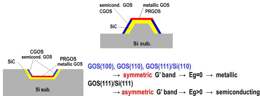
図 4.1.10 μGOS 技術。メサエッチングによる微小領域への選択的 GOS 形成。エッチングで現れる複数の面方位により、多層化グラフェンの積層様式・電気的特性が異なり、バンドギャップ発現による On/Off 比向上に必要な CGOS と単層グラフェンのギャップレス・線形分散特性が必要な PRGOS の作り分けが可能。
