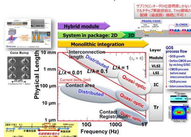
図 4.1.13 Si-CMOS と完全整合する CGOS/PRGOS-CMOS プロセス技術の実現。
