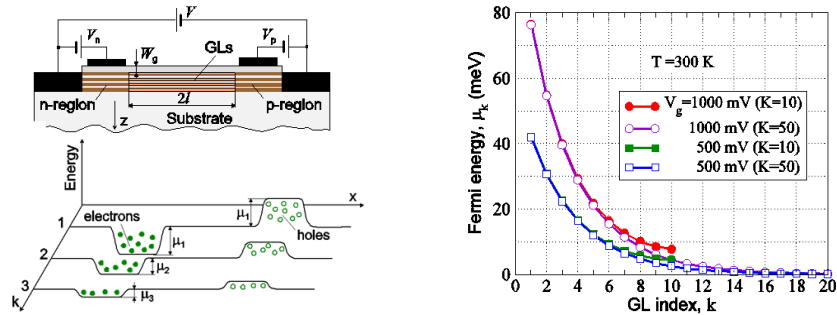
図 4.3.3 左：多層グラフェン FET におけるトップゲート制御性の模式図[34]、右：トップゲート電圧印加時におけるフェルミ準位の層依存性[34]。
