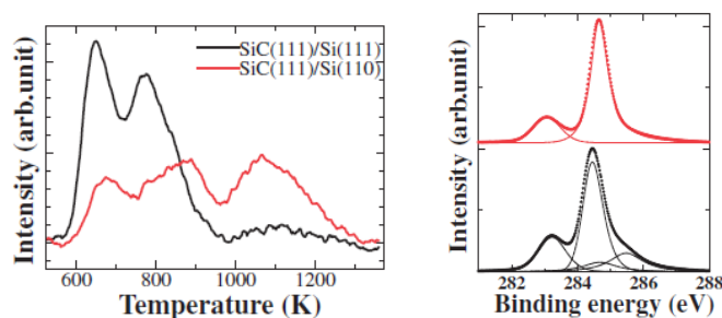
図 4.1.7 左: 3C-SiC/Si 表面からの D 2 -TPD スペクトル。SiC(111)/Si(111)表面からのスペクトル(黒)は C-D ピークが弱く Si 終端であることを示すのに対し、SiC(111)/Si(110)表面からの TPD スペクトル(黒)は C 終端 3 \times 3 構造特有の強い C-D ピークを示し、表面が C 終端になっていることを示す。右: C1s-XPS スペクトル。SiC(111)/Si(111)表面からのスペクトル(下)は界面層の存在を示すピーク(285.5 eV)を示すが、SiC(111)/Si(110)表面はこれを示さない。
