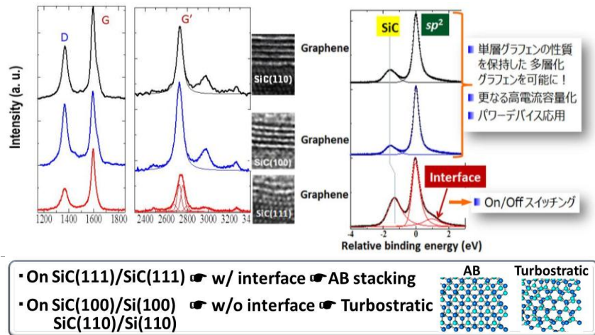
図 4.1.8 Raman スペクトル, TEM, XPS による GOS の基板面方位に対する積層様式の依存性。
