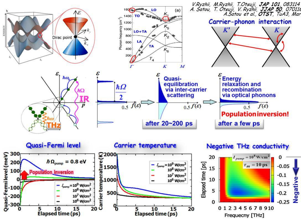
図 4.3.6 グラフェンのバンド分散特性、フォノンバンド図、光学フォノン散乱（以上は左上から右上の順）、光学励起グラフェンのキャリアエネルギー緩和の様子（中段）、赤外線レーザーによるインパルスポンピング後の電子疑似フェルミ準位（左下）、キャリア温度（中下）、および導電率（右下）の時間発展解。ポンピングによってキャリア温度が一気に上昇するが光学フォノンの放出によるエネルギー緩和によってキャリア温度は急速に低下し、それとともなって、疑似フェルミ準位が上昇し一定のポンピング強度以上では 10ps 以上の時間にわたって正値（反転分布）を保つ。その結果、ポンピングから 2ps 程度の内に、導電率は広いテラヘルツ帯で負値になり、10 p s オーダの時間スケールで平衡状態へと推移する。[53, 69, 70, 76-78]
