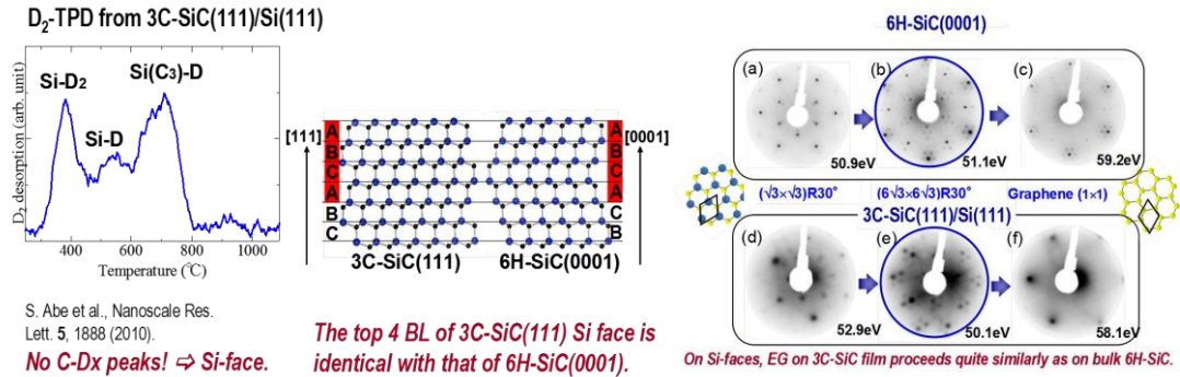
図 4.1.5 3C-SiC(111)/Si(111)表面からの D 2 -TPD スペクトル(左)。C-D ピークが弱く Si 終端面であることがわかる。Gr/3C-SiC(111)の Si 面では、6H-SiC(0001)面と最上層 4 層分は同一の構造を有する(中)。LEED 観察像の比較 (右)。グラフェン形成後(右端)においては極めて類似の構造を有する。
