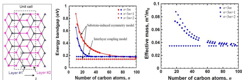
図 4.4.1 強束縛法によるバイレイヤーグラフェンのエネルギーバンド、有効質量計算結果[22]。
