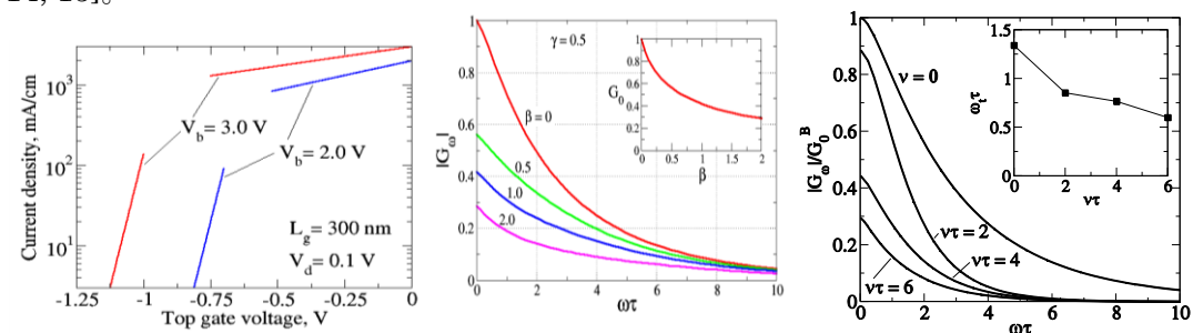
図 4.3.1. グラフェンナリボンチャンネル FET (左、中) における動作特性。左：DC ドレイン電流のゲートバイアス依存性[4]、中：AC トランスコンダクタンスの周波数依存性（挿入図は DC トランスコンダクタンスの電子衝突パラメータ依存性）[7]、右：二層グラフェンチャンネルFET におけるACトランスコンダクタンスの周波数依存性[15]。
