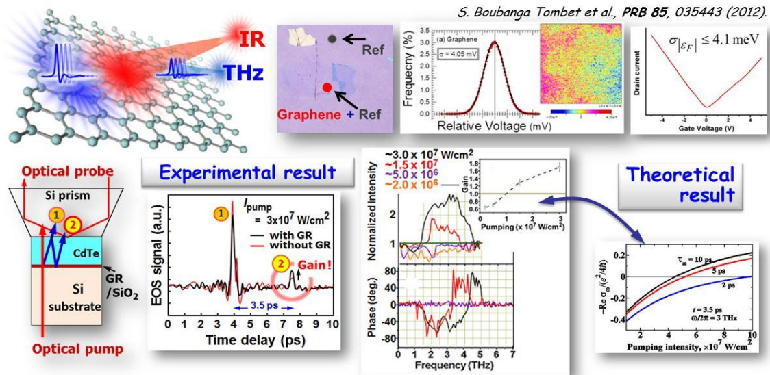
図 4.2.11 フェムト秒 IR レーザーによる光学励起グラフェンからの THz 誘導放出。実験のイメージ（左上）、被測定剥離グラフェンの光学顕微鏡像、ケルビンプローブによる表面ポテンシャル分布像、Dirac 電位がほぼ 0V のアンバイポーラ特性（以上は右上）、実験系、時間応答波形、利得スペクトルのポンピング閾値特性、ポンピング閾値特性の数値解析結果（以上は左下から右下の順） [66]。
