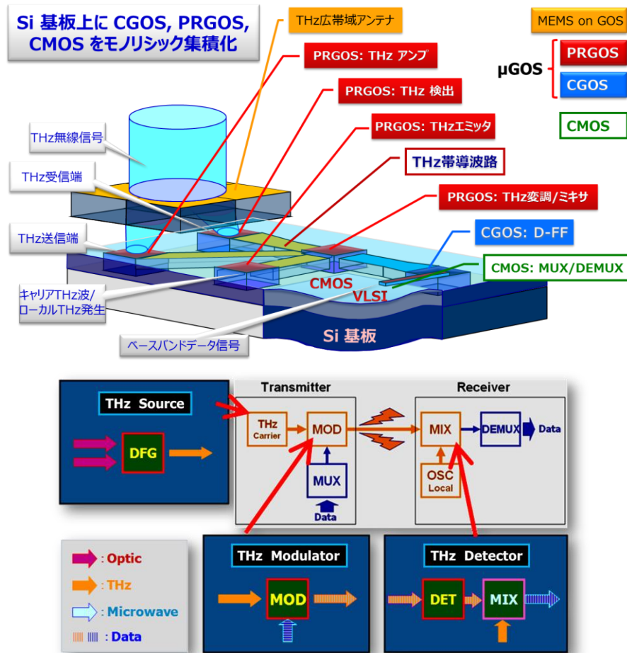
図 8.3 超高周波テラヘルツ無線通信トランシーバフロントエンドの GOS による 1 チップ化イメージ。
