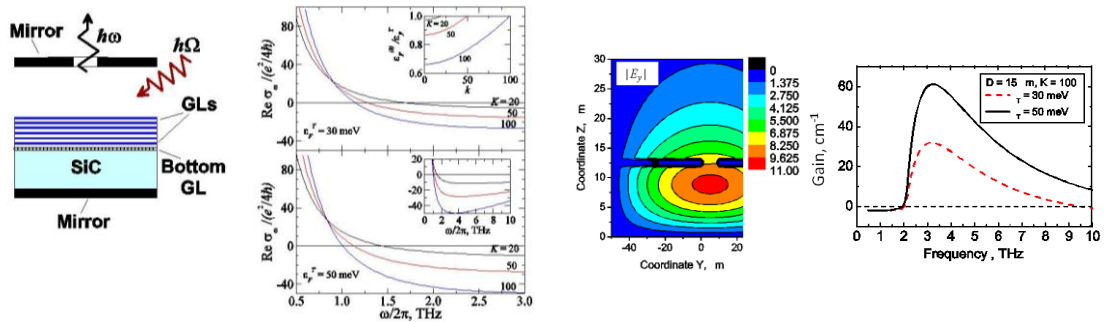
図 4.3.7 左：多層グラフェンを用いた縦型共振器レーザーの光ポンプ時における伝導率の周波数依存性（ K はグラフェン層数、 \epsilon_F は最上層における擬フェルミエネルギー）[20]。右：スロットライン絶縁体導波路組み込み型多層グラフェン THz レーザーにおける、放射 THz 波強度分布と光ポンプ時における出力周波数－利得係数特性 [27]。
