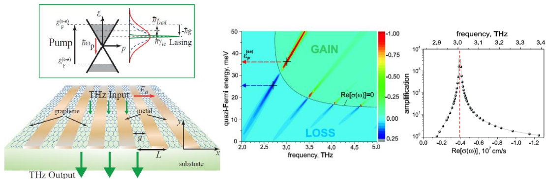
図 4.3.10 金属回折格子を設置したグラフェンの表面プラズモンポラリトンによるテラヘルツ帯巨大利得増強作用 [80]。
