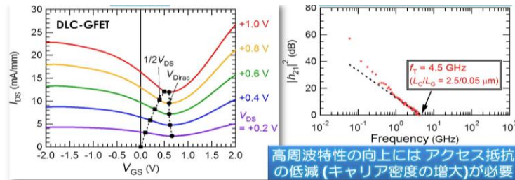
図 4.2.5 DLC をゲート絶縁膜に導入したグラフェンチャネル FET の伝達特性 (チャネル長 6\ \mu\text{m} 、ゲート長 5\ \mu\text{m} ) [65]と電流遮断周波数特性 (チャネル長 2.5\ \mu\text{m} 、ゲート長 50\ \text{nm} )。
