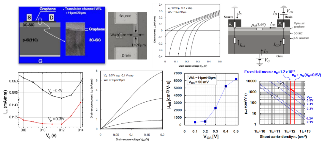
図 4.2.1 バックゲート型 GOSFET。上左：GOSFET 断面・上面写真、上中：基板リークを含むドレイン電流・電圧特性[29]。上右：基板リークパスを含む GOSFET 等価回路モデル。左下：アンバイポーラ特性[30]、左
