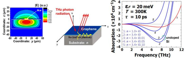
図 4.3.9 光学励起によって反転分布状態におかれたグラフェンに励起された表面プラズモンのテラヘルツ帯利得増強効果。テラヘルツ帯導波路は放射損と自由キャリア吸収が大きく低損失化が困難であり、量子カスケードレーザでも高温動作化の障壁となっている。本成果はその導波路自体に巨大利得増強効果が得られることを示したものの。[39]
