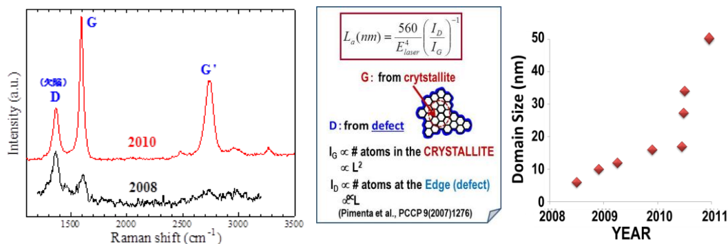
図 4.1.4 研究当初(2008 年)と現在(2010 年)のグラフェンの Raman スペクトルの比較。欠陥密度が 90%低減されたことが、D バンドと G バンドの強度比から明らかとなった。G' バンドの強度が強くなったことは、グラフェンの二次元結晶性が飛躍的に向上したことを示唆する。
