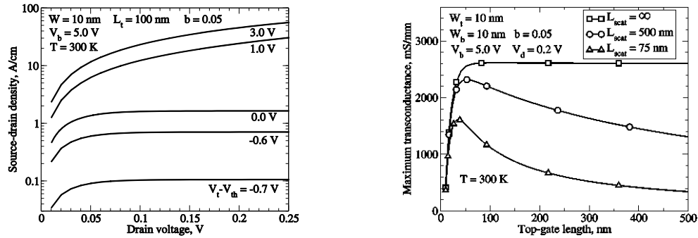
図 4.3.2 左：二層グラフェン FET における電流－電圧特性[36]、右：最大トランスコンダクタンスのトップゲート長依存性 [36]。
