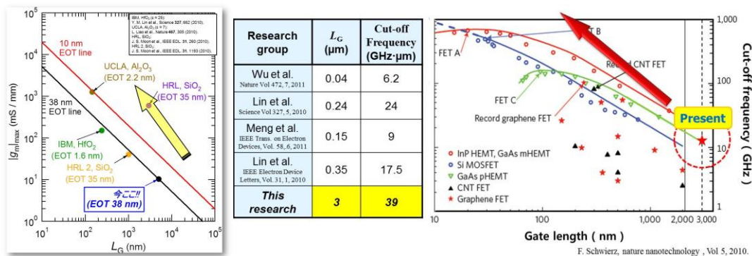
図 4.2.12 左上：Gm のスケーリング予測。右上：ft のスケーリング予測。
