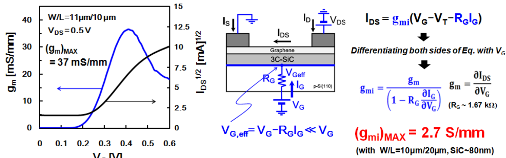
図 4.2.2 バックゲート型 GOSFET の相互コンダクタンス:gm。左：実測値、右：等価回路モデルによる真性 FET 領域の相互コンダクタンス:gmi の抽出[32]。
