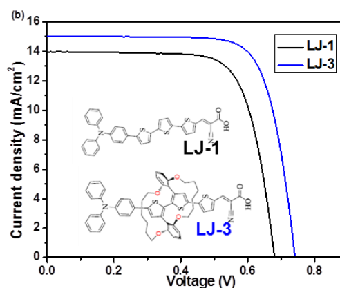
図6 新規色素とそのI-V曲線
