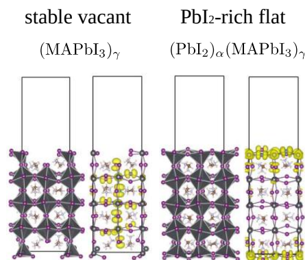
図 24 \text{CH}_3\text{NH}_3\text{PbI}_3 の安定な表面終端構造。 準安定の左者がホール受容状態を表面にもつ
