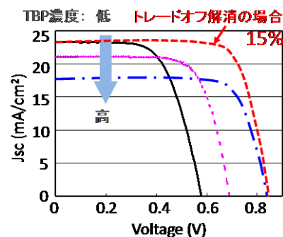
図 29 TBP 添加におけるトレードオフ
