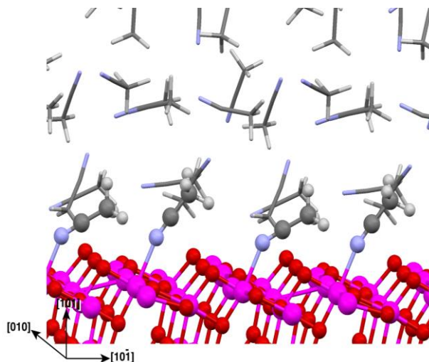
図 21 \text{TiO}_2(101) /アセトニトリル溶液界面の計算結果
