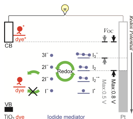
図 23 アセトニトリル溶媒中のI-/I 3 -レドックス反応中間状態の酸化還元電位
