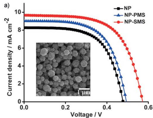
図2 \text{SnO}_2 粒子を用いたセルの特性(NP: ナノ粒子、SMS: 400nmの階層構造)
