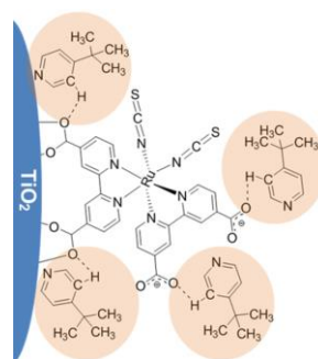
図 16 \text{TiO}_2 上の N719 色素と TBP の相互作用の模式図
