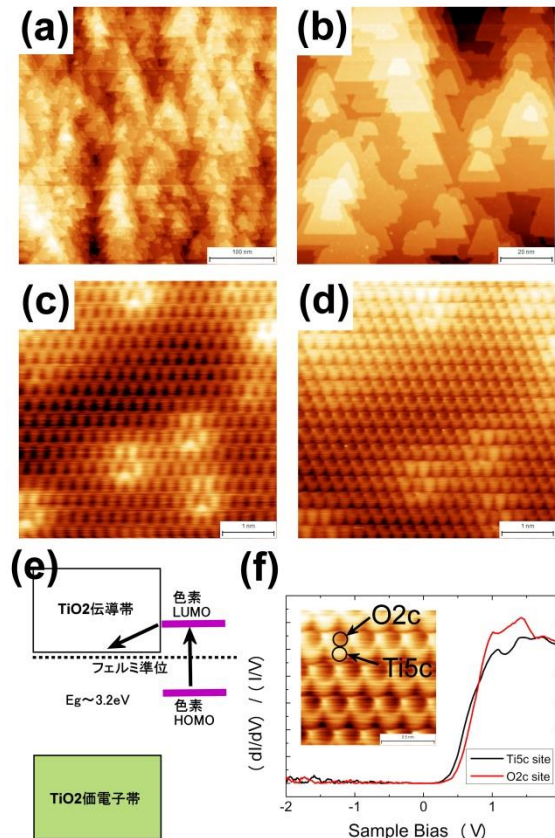
図 19 (a)(b) TiO 2 アナターゼ (101) 表面の STM 像.イメージサイズ:(a) 400nm×400nm, (b)100nm×100nm, サンプルバイアス: +2.0V, トンネル電流: 0.1nA, 試料温度:78K, (c)(d) 原子分解能 STM 像, イメージサイズ=5nm×5nm, サンプルバイアス: +1.0V, トンネル電流: (c)0.4nA, (d)2.0nA, 試料温度:78K, (e) TiO 2 と色素分子のバンド図, (f) アナターゼ表面の規格化トンネルスペクトル.
