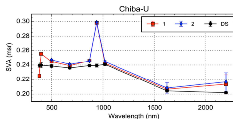
図3.3-3 ディスクスキャン法(Disk scan (DS); SKYNETで採用されている方法)と積分球から求めた直達光に対する校正定数(立体視野角, SVF)の比較。1はBaSO 4 , 5.8 A(150 W)×4の積分球を, 2はBaSO 4 , 4.8 A(150 W)×4の積分球を使用した結果である。DSはディスクスキャン法による結果である。
