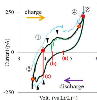
図 7 Bundle-NW 電池の CV 曲線、黒三角印は 4\ \text{V} 反応の Double peak。丸数字は図 7 の TED 観察時点で、丸アルファベットは図 8 (a), (b), (c) の TED 観察時点である。
