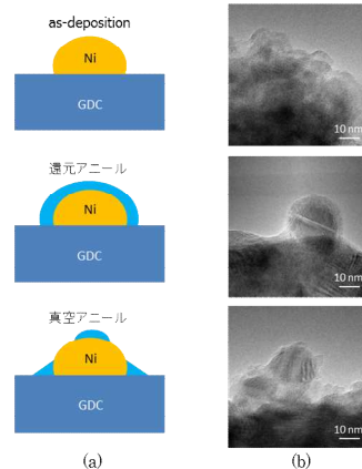
図 30 (a) モデル触媒を用いた SMSI 効果検証実験の模式図(b)それぞれの段階に対応した TEM 像。試料アニール: 500—1000℃, 2-3h
