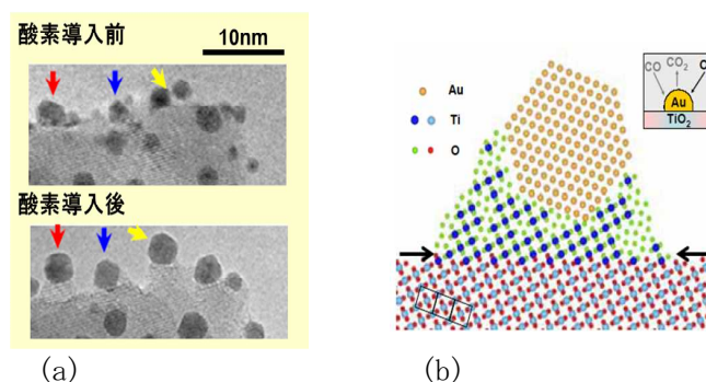
図 20 (a) \text{Au/TiO}_2 試料と酸素ガス ( 100\text{Pa} ) を導入する前と導入した後の TEM 像、(b) 酸素ガスと \text{Au/TiO}_2 界面周縁に形成された \text{Ti}_{1-x}\text{O}_2 相の模式図
