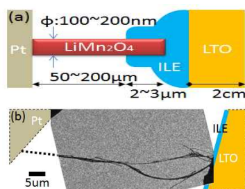
図 5 Bundle-NW 電池 (a) 構成、 (b) TEM 写真
