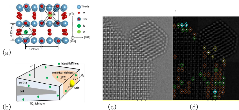
図 19 (a) \text{TiO}_2 (ルチル型) 結晶と格子間チタンイオンの模式図. (b) TEM 観察した楔形チタニア基板と付着した金ナノ粒子との周辺に形成される Ti イオンの欠損域模式図. (c) \text{TiO}_2 結晶の高分解能 TEM 写真と格子間チタンイオンの像. チタニア試料の端部に見える格子間チタンイオンを矢印で示す. (d) 金粒子とチタニア界面の縁に周集積した格子間チタンイオン. ならびに、チタニア基板内に分布している格子間チタンイオン. 格子間チタンイオンが見える場所を、オレンジ、緑、青色の菱形図形で示してある。
