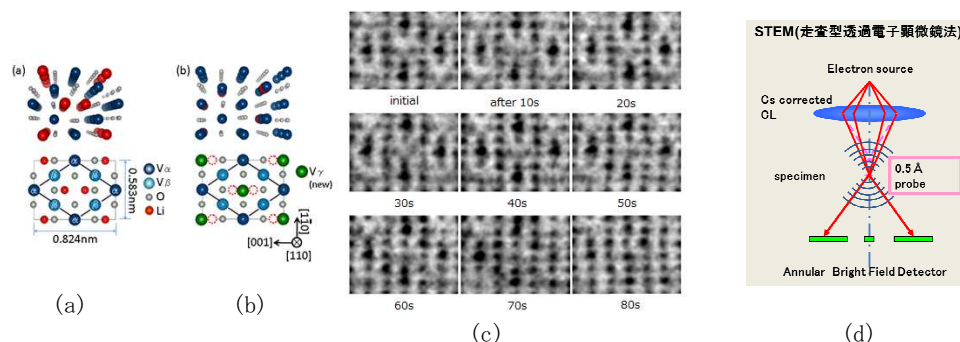
図 18 50pm 分解能電子顕微鏡による \text{LiV}_2\text{O}_4 結晶 “その場” 観察. (a) [110] 方向から見たスピネル構造模式図. (b) defective-NaCl 構造の模式図. (c) \text{LiV}_2\text{O}_4 結晶構造変化を示す ABF 像シリーズ. ABF 像のカラム強度変化は、Li イオン(赤色)が 4 面体位置から移動した結果、V イオン(青色)の移動が誘起されていることを示した. (d) ABF (環状明視野像) の観察方法の概念図.
