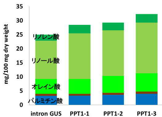
図2. PPT遺伝子を過剰発現したダイズの脂肪酸組成
