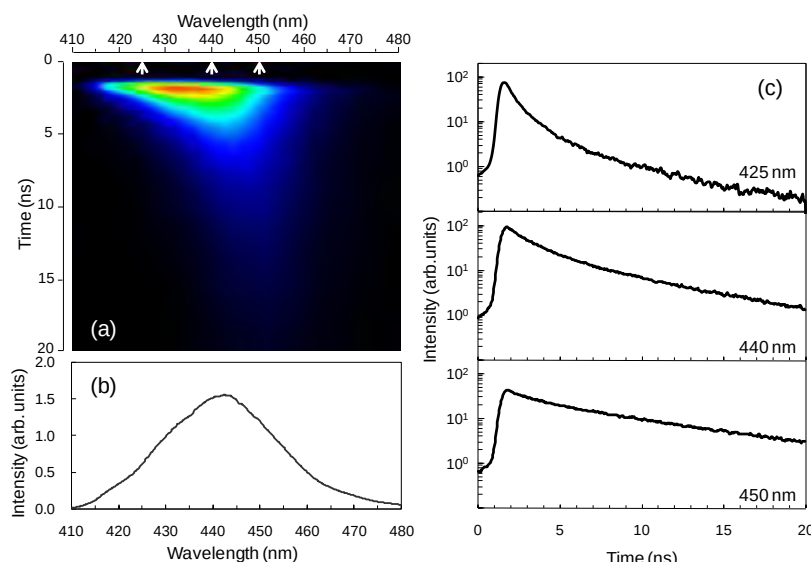
図 16 近紫外線ピコ秒パルス光源を励起源としてストリークカメラによりサファイア基板上に成長した InGaN-SQW 構造の時間分解 PL 分光測定を行った結果. (a) 時間分解のスペクトログラム, (b) 時間積分した PL の発光スペクトル, (c) 異なった 3 つの波長成分で見た PL の時間的变化.
