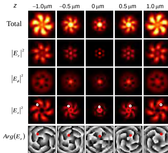
図13 らせん状位相分布を持つ二つの径偏光ビームを合波した場合の焦点前後での強度、偏光および位相分布の変化の例。
