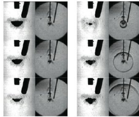
図 14 圧力波（衝撃波）の伝播
