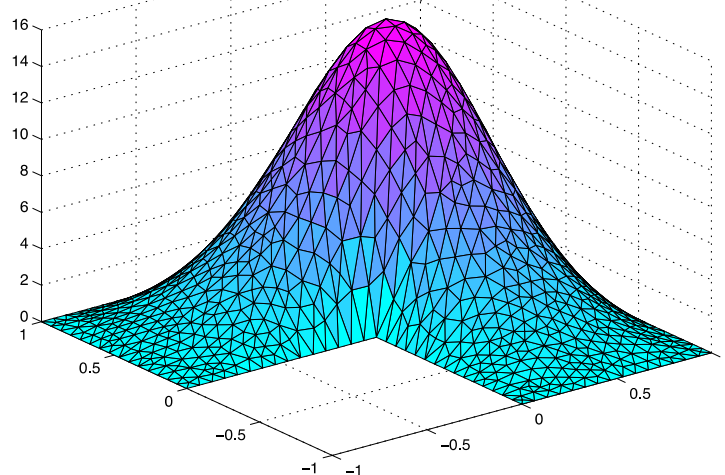
図 3. L 字領域上での Emden-Fowler 方程式の数値解
