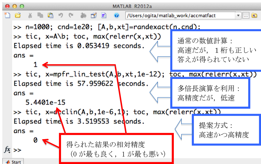
図13: 高精度行列分解アルゴリズムによる悪条件線形方程式の高精度数値計算結果
