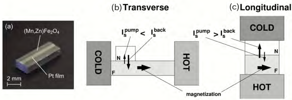
図 18 : (a)縦型スピントラック効果の試料写真。(b)横型スピントラック効果の概略図。(c)縦型スピントラック効果の概略図。
