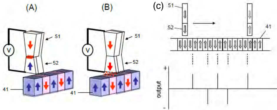
図10: スピン起電力再生ヘッド。(A)磁化が固定された磁化固定部 51 と、磁化固定部に接合され外部磁界によって磁化が変化する磁化自由部 52 と、磁化固定部と磁化自由部にそれぞれ接続された一対の出力端子から構成される。磁化固定部と磁化自由部の接合部のくびれで磁壁(波線)をトラップする。(B)磁化自由部中の磁壁の移動に伴うスピン起電力を用いて外部磁界の変化を検出する。(C)スピン起電力再生ヘッドの作動例と出力信号シーケンス。
