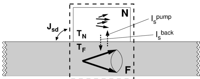
図 16 :スピントラック効果の微視的メカニズム。磁性体(F)内の局在磁化が熱揺らぎによりスピンホール電極(N)内にスピンドラッグを注入する。
