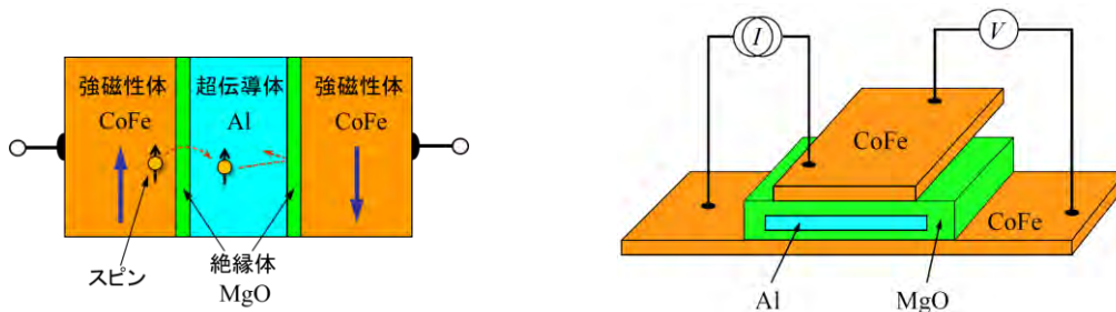
図25：二重トンネル接合デバイスの概念図(左図)。左右の強磁性電極(CoFe)の磁化の向き(青色矢印)を互いに反平行の配置にすることで、スピンを超伝導体に注入し、長い時間保持することができる。今回、作成した二重トンネル接合デバイスの構造(右図)。
