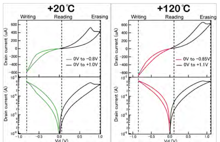
図19 無電解金メッキにより作製したナノギャップ電極の負性微分抵抗を含む電流-電圧特性(左:常温, 右: 120^{\circ}\text{C} )
