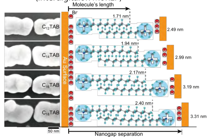
図4 CnTAB を界面活性剤として用いた MoREP により作製したナノギャップ電極の SEM 像と概念図
