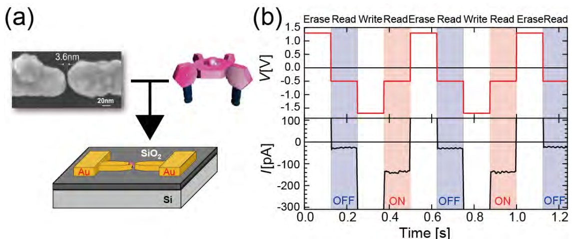
図17 (a) 固体基板上分子メモリの模式図、(b) 固体基板上における室温単分子メモリ効果
