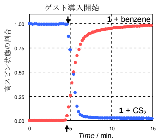
図 2-7 1 のゲスト雰囲気下におけるスピン状態変化
