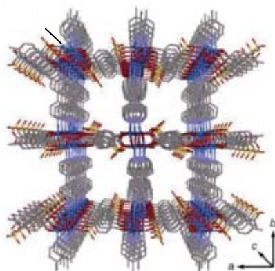
図 2-1 [Zn 3 (μ 3 -OH) 3 (2-stp)(bpy) 1.5 (H 2 O)] の構造
