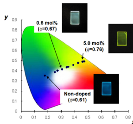
図 1-8 有機シリカ薄膜における色素導入量による発光色制御
