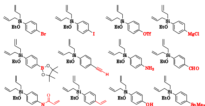
図 2-1 種々のアリルシリルゾル・ゲル前駆体(MBAS)
